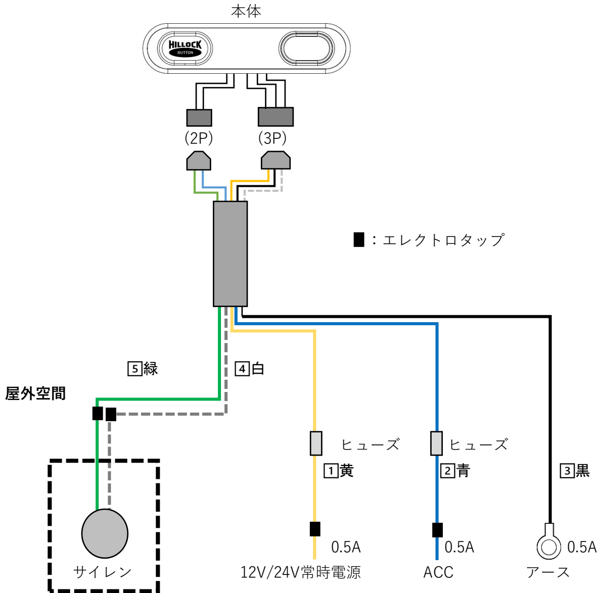
接続全体図(OSB-100)
